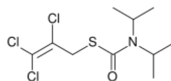
Strukturformel von Triallat
