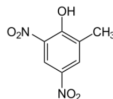
Strukturformel von Dinitroorthokresol
